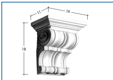
CARTEL·LA ONDULADA
