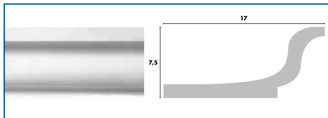
LLUM INDIRECTE SAFATA
