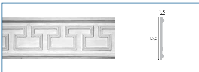
FRISOS 110
