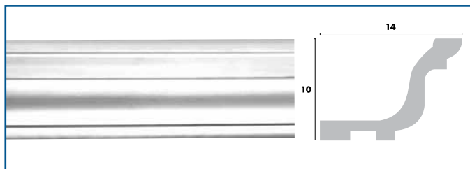
LLUM INDIRECTE N. 14
